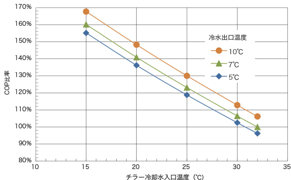
図2. 冷却水温度と COP (スクリーチャー R134a)
