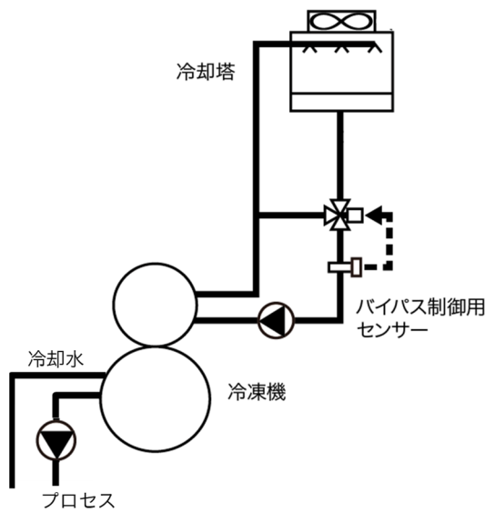
図 1. 冷却塔のバイパス制御
