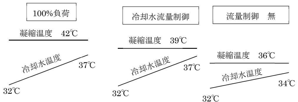
図 3. 低負荷（負荷率 40%）時の冷却水流量制御と凝縮温度の関係
