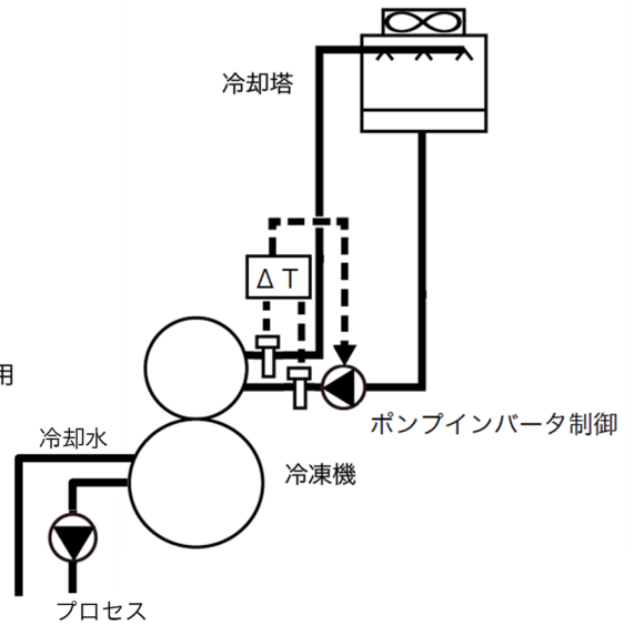
図 2. 冷却水流量制御
